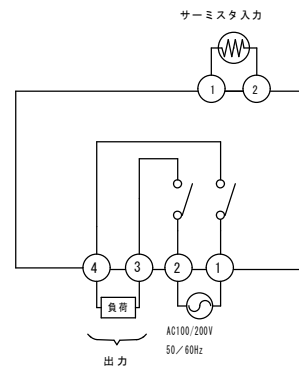
端子接続図
