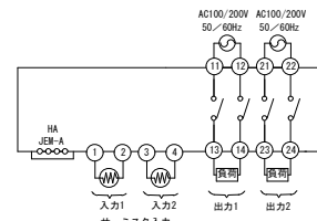
端子接続図
