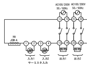
端子接続図
