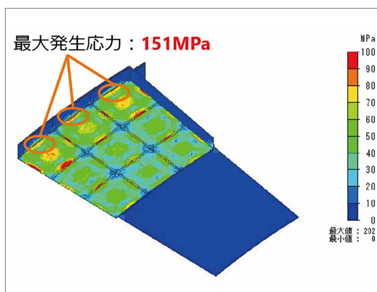
応力分布図
