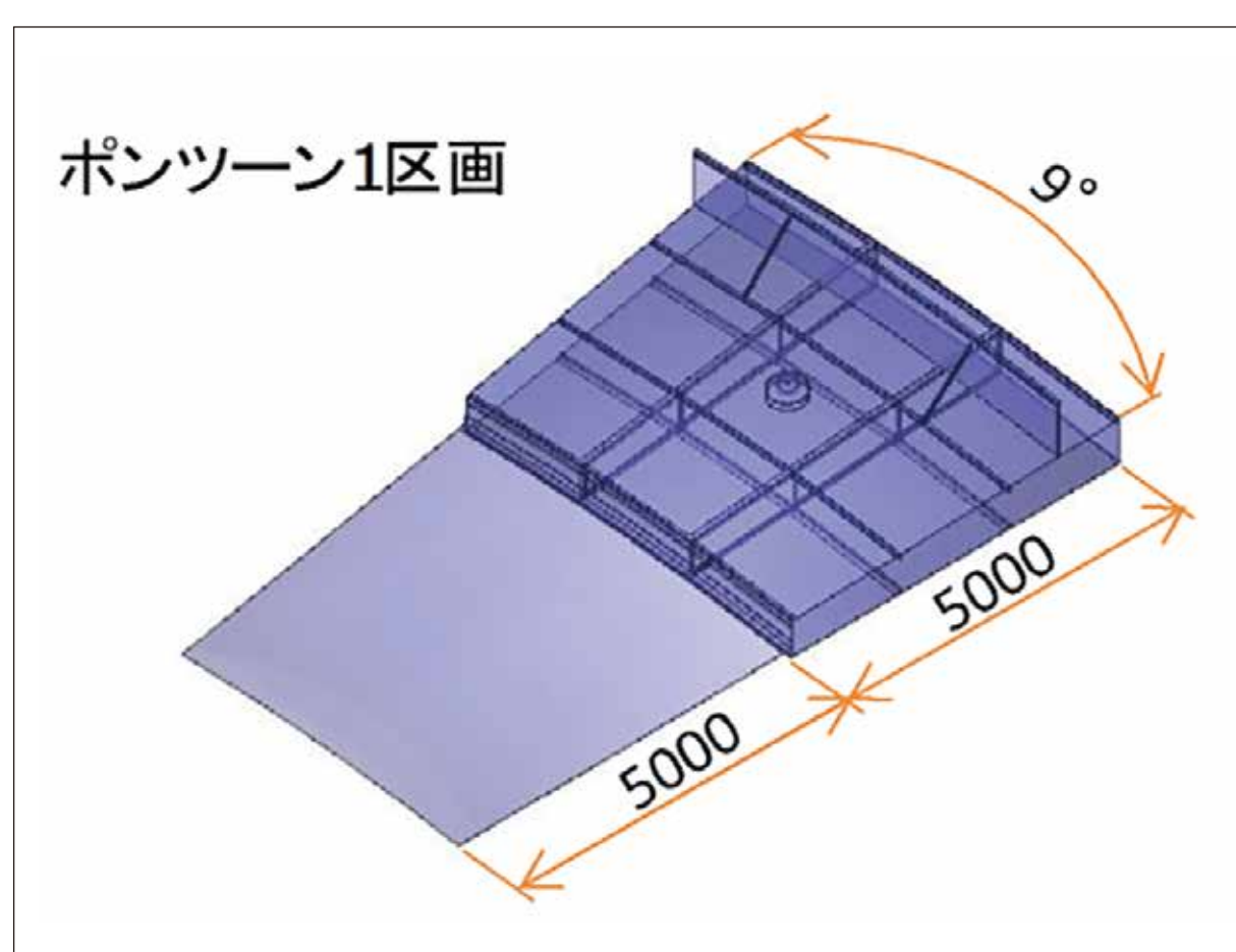
浮き屋根タンクポンツーンモデル
