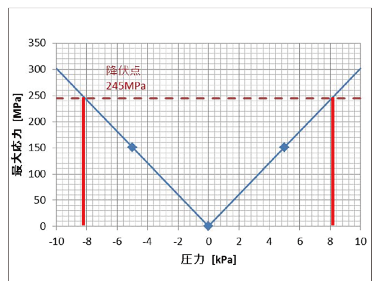
内圧と最大応力関係
