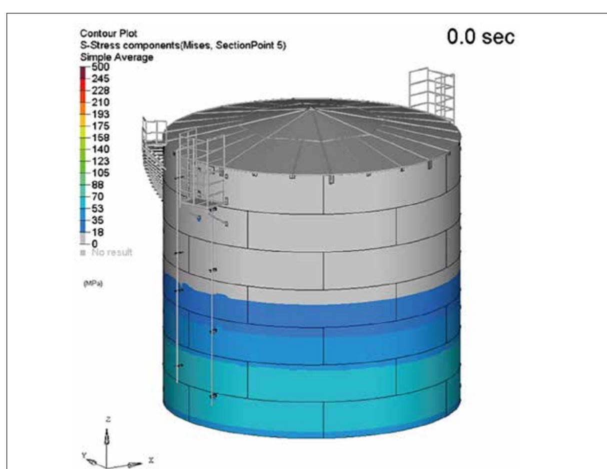
タンク解析モデル図
