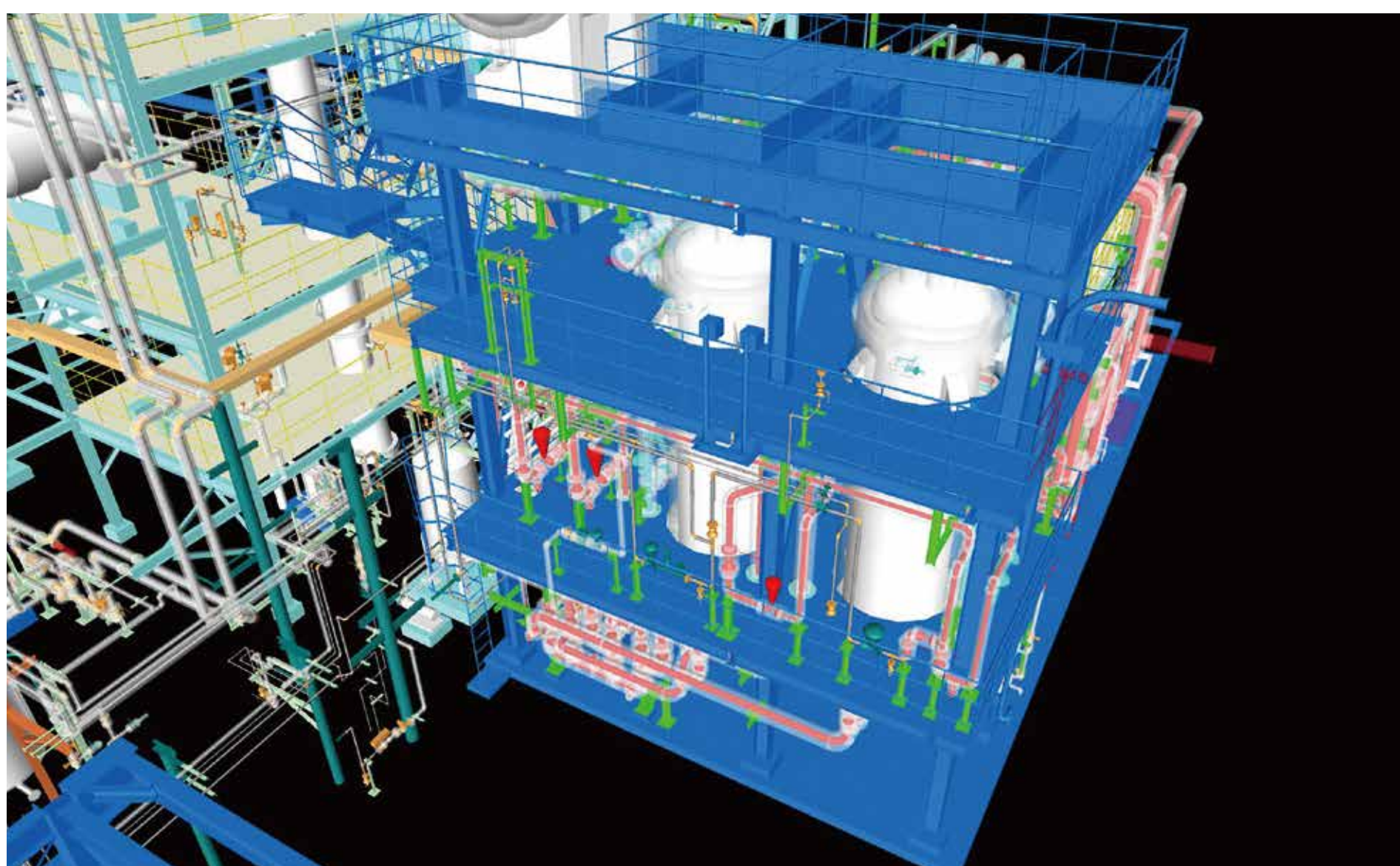
新設範囲3D CADデータ
