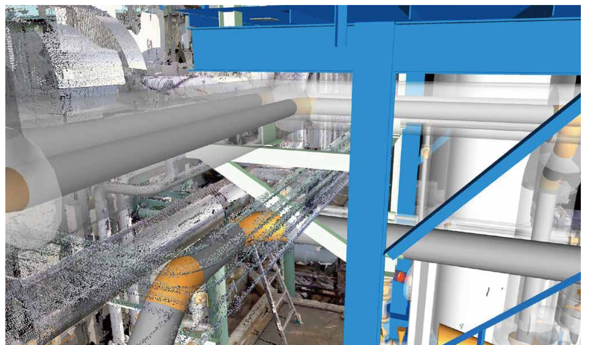
レーザー計測点群データと3D CADデータの干渉確認
