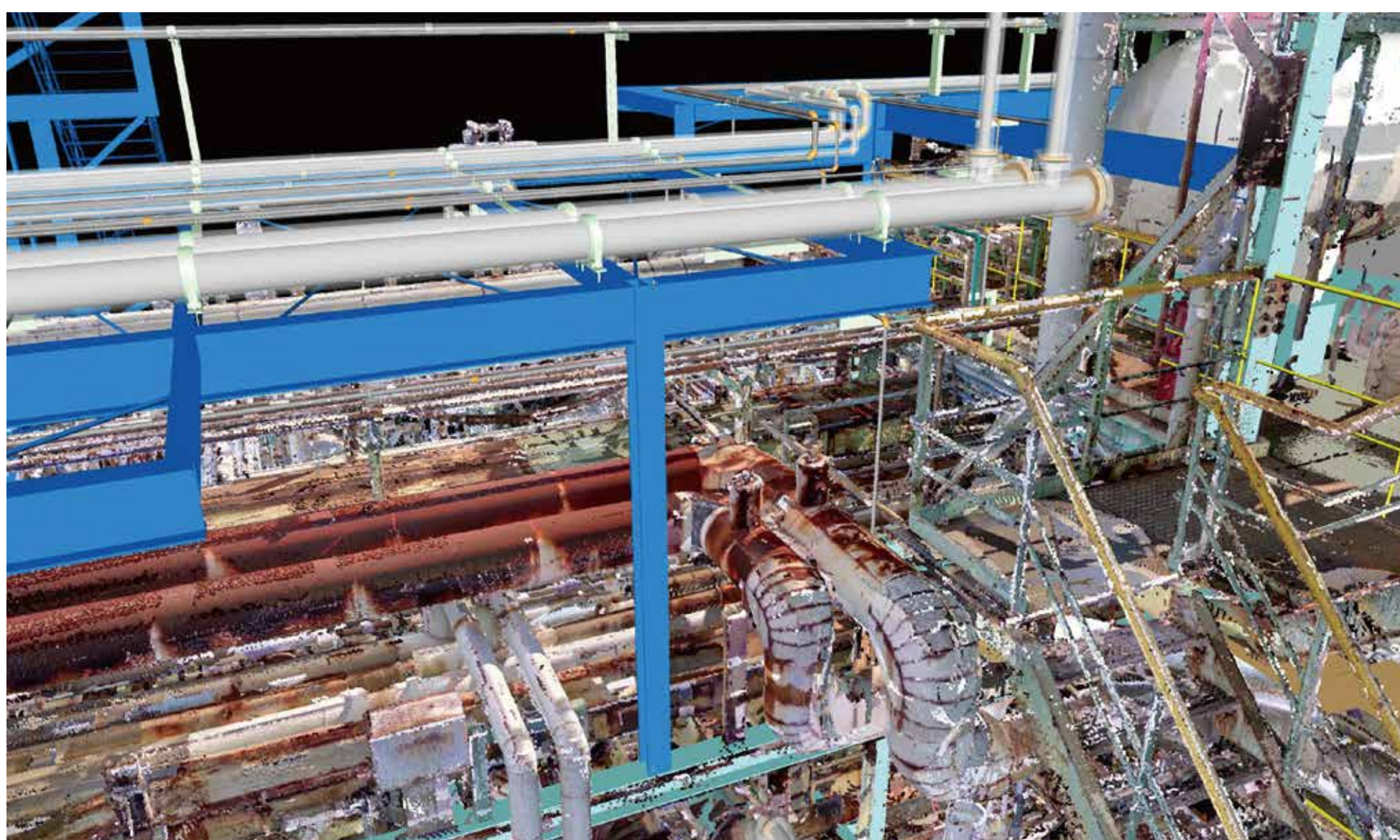
レーザー計測点群データと3D CADデータの干渉確認
