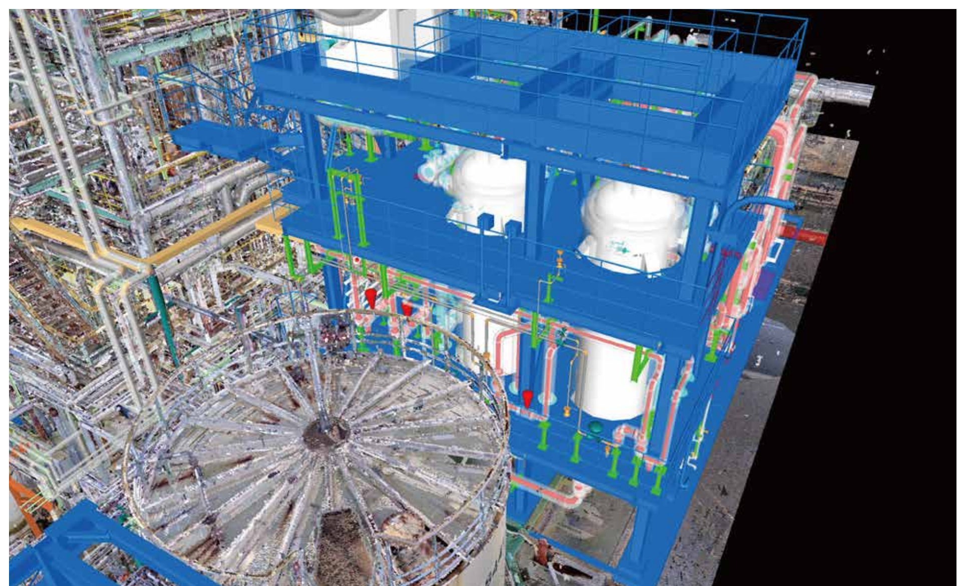
レーザー計測点群データと3D CADデータを合成
